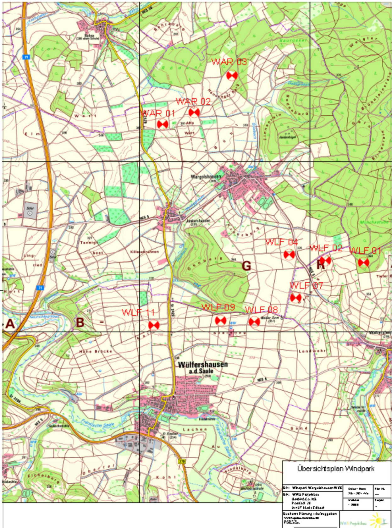
Abbildung: Übersichtslageplan. Die Windenergieanlagen WLF 1, 2, 4, 7 und 8 werden von der Emittentin betrieben. Die übrigen Windenergieanlagen werden planmäßig von der Bürgerwindenergie Weißer Turm Nord GmbH & Co. KG betrieben.
